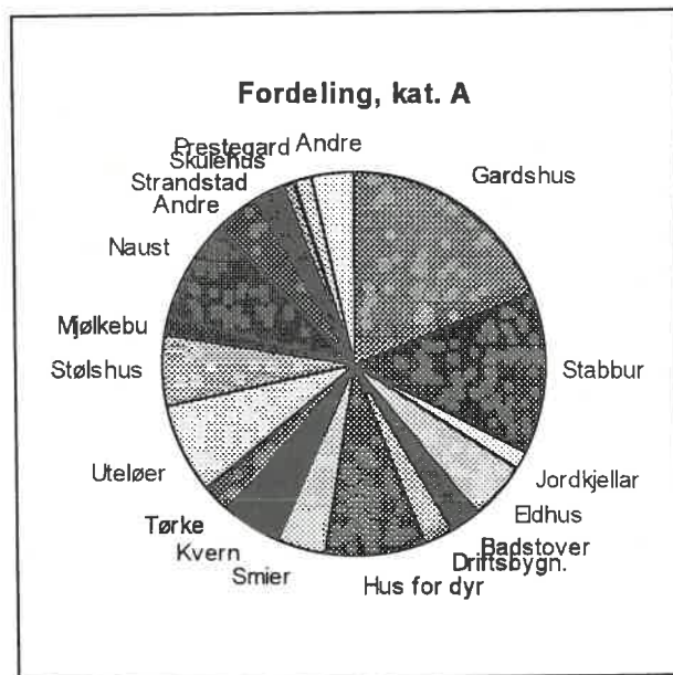
Fig. 4 Fordeling, kategori A.
