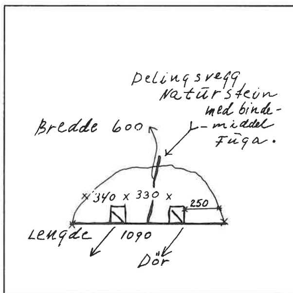
Snitt gjennom jordkjellar, Bjørklund etter teikning av Jarleiv Bjørklund.
